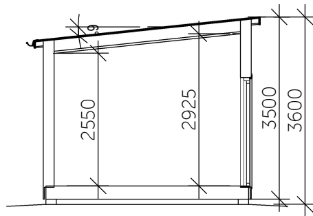
SEKTION A-A
