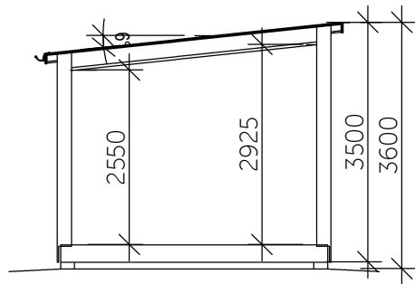
SEKTION A-A
