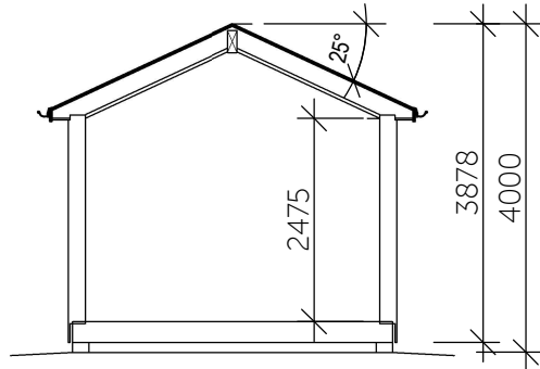
SEKTION A-A
