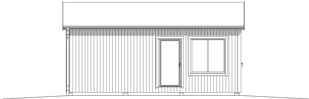
Fasad 3
