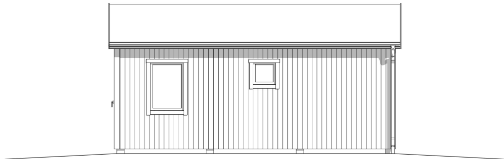
Fasad 1
